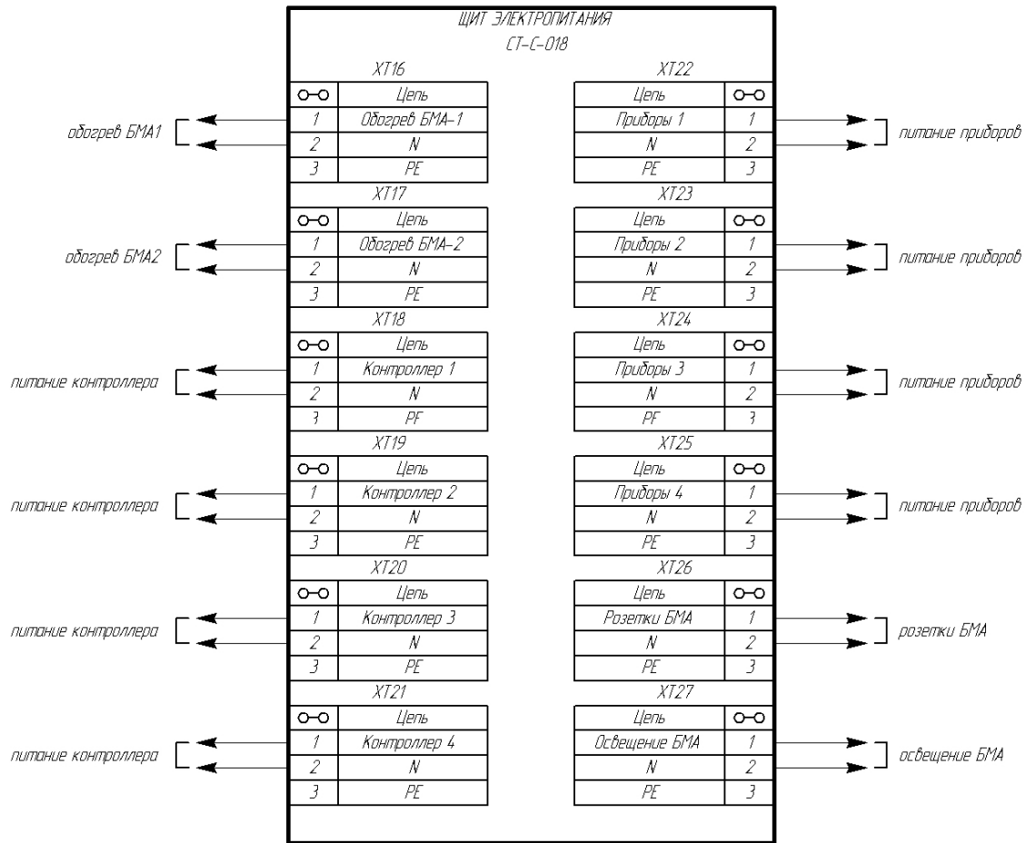
Рисунок 3 - Схема подключения однофазных силовых нагрузок
