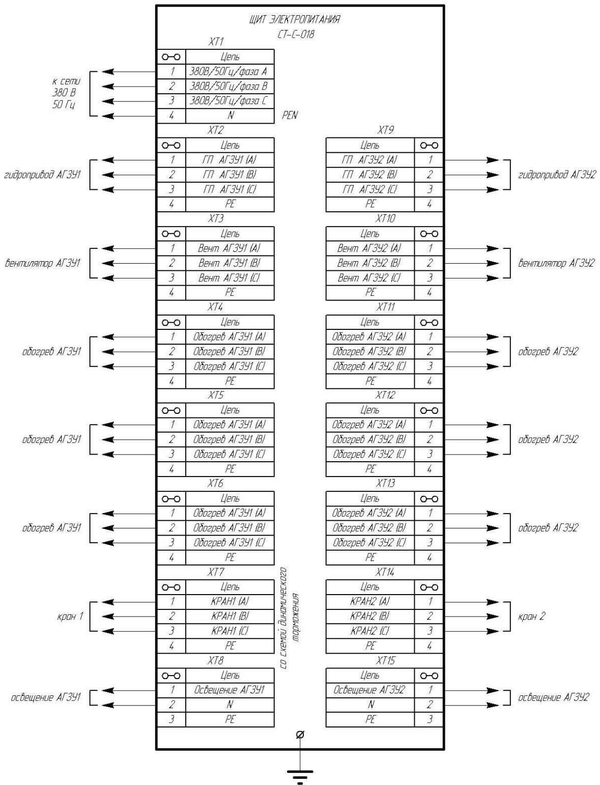
Рисунок 2 - Схема подключения трехфазных силовых нагрузок
